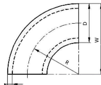
Oblouk | Elbow | Колено 90°
