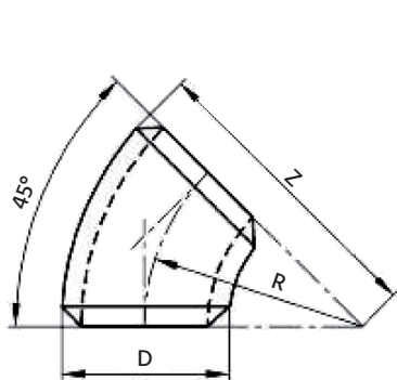
Oblouk | Elbow | Колено 45°
