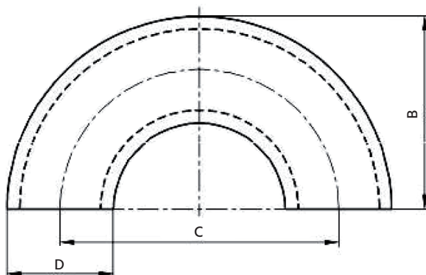
Dvojitý oblouk | Double elbow | Двойное колено 180°
